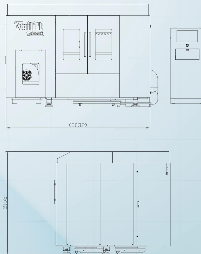
TL-1515C 佔地面積圖
